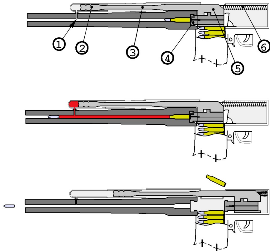
(cc) Thuringius - Funktionsprinzip eines Gasdruckladers
